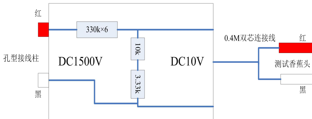
图 1 DC1500V/DC10 变换器电气原理图
